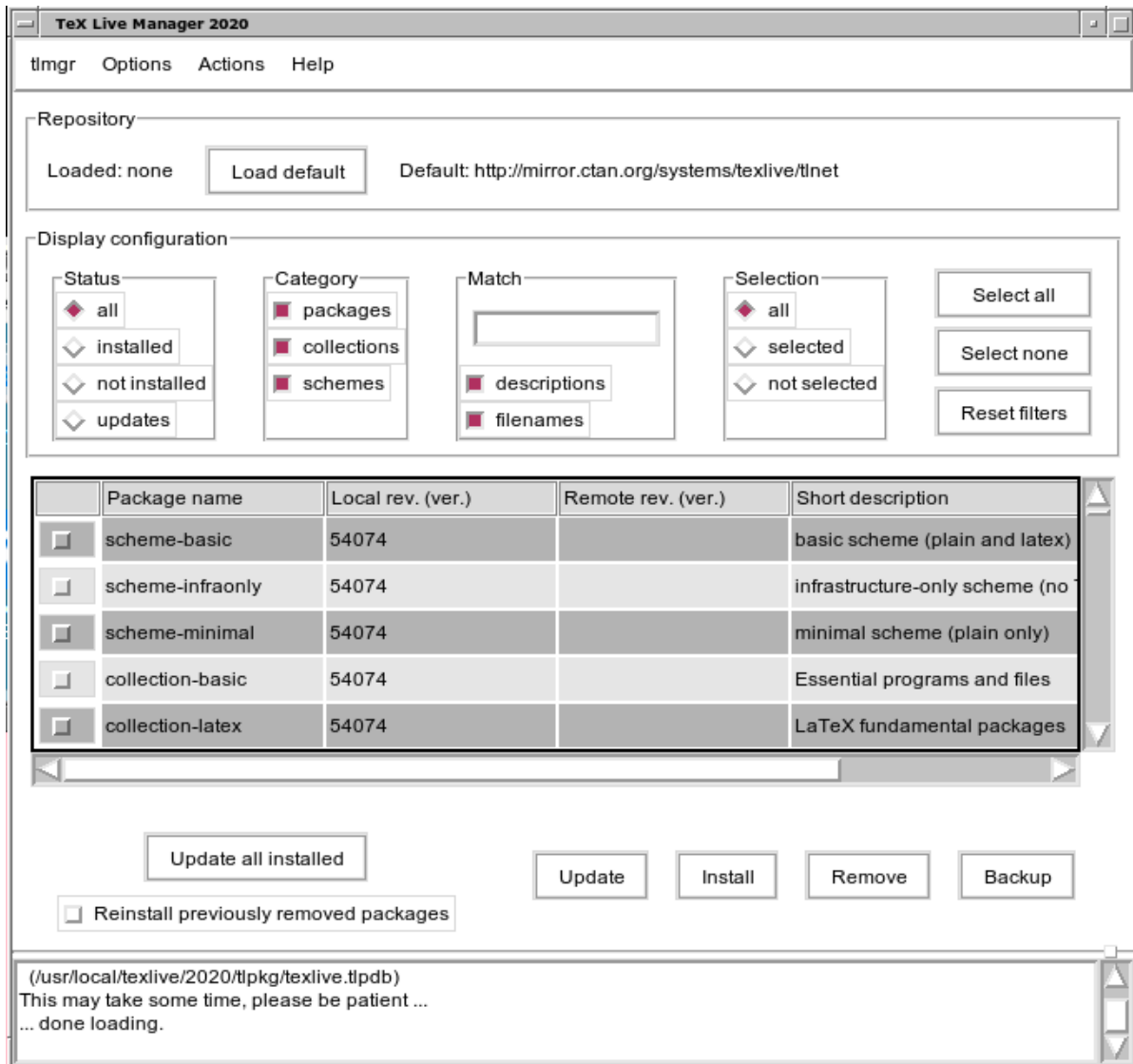
FIGURE 11 – Ancien mode GUI pour tlmgr : fenêtre principale, après « Chargement »
